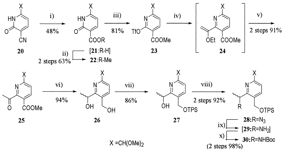
Scheme 2. Reagents and conditions: i) 6 M KOH, EtOH, reflux, 8 h, 0 °C, 30 min, rt, 2 h, ii) \text{H}^+ , MeOH, reflux, overnight, iii) \text{Tf}_2\text{O} , DMAP, pyridine, 0 °C, 30 min, iv) \text{Pd}(\text{OAc})_2 , dppp, ethyl vinyl ether, v) 70% AcOH, THF, rt, overnight, vi) \text{NaBH}_4 , \text{CaCl}_2 , EtOH, 0 °C, 30 min, rt, 3 h, vii) TPS-Cl, \text{Et}_3\text{N} , DMAP, \text{CH}_2\text{Cl}_2 , 0 °C, 30 min, rt, 2 h, viii) a) \text{MsCl} , \text{Et}_3\text{N} , \text{CH}_2\text{Cl}_2 , 0 °C, 10 min, b) \text{NaN}_3 , DMF, rt, 1 h, ix) \text{H}_2 , 10% Pd-C, EtOH, rt, 30 min, x) \text{Boc}_2\text{O} , \text{Et}_3\text{N} , \text{CHCl}_3 , 0 °C, 30 min, rt, 4 h.
