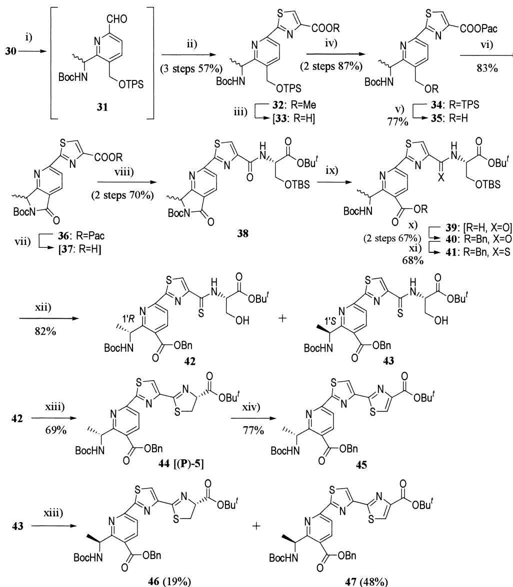
Scheme 3. Reagents and conditions: i) 2 M HCl, rt, overnight, ii) a) HCl·H-L-Cys-OMe, Et 3 N, toluene, rt, 10 h, b) MnO 2 , toluene, rt, overnight, iii) 1 M LiOH, H 2 O–dioxane (1:1 v/v), 0 °C, 30 min, rt, 8 h, iv) PacBr, Et 3 N, DMF, 0 °C, 30 min, rt, 6 h, v) TBAF, THF, 0 °C, 30 min, vi) Jones reagent, acetone, 0 °C, 30 min, rt, 8 h, vii) K 2 CO 3 , THF, H 2 O, 0 °C, 30 min, rt, 8 h, viii) H-L-Ser(TBS)-OBu t , DPPA, Et 3 N, DMF, 0 °C, 30 min, rt, overnight, ix) 1 M LiOH, THF, H 2 O, 0 °C, 30 min, rt, 1 h, x) BnBr, Et 3 N, DMF, 0 °C, 30 min, rt, 12 h, xi) Lawesson's, reagent, DMF, 50 °C, 12 h, xii) 2 M HCl, THF, rt, xiii) Ph 3 P, EDAD, THF, 0 °C, 30 min, xiv) MnO 2 , toluene, rt, 20 h.
