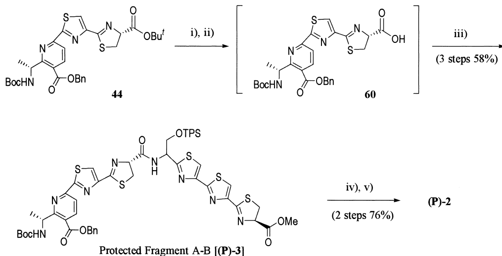
Scheme 6. Reagents and conditions: i) THF-CHCl 3 (3:2 v/v), rt, 5 h, ii) Boc 2 O, Et 3 N, CHCl 3 , 0 °C, 30 min, 5 h, iii) (P)-4, BOP, ( i -Pr) 2 NEt, DMF, 0 °C, 30 min, rt, 4 h, iv) TFA-CHCl 3 (2:3 v/v), rt, 30 min, v) (P)-6, BOP, ( i -Pr) 2 NEt, DMF, 0 °C, 30 min, rt, 12 h.
