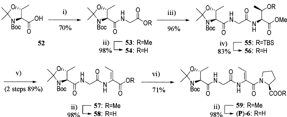
Scheme 5. Reagents and conditions: i) DCC, HOSu, HCl·H-Gly-OMe, CH 2 Cl 2 , 0 °C, 30 min, rt, 6 h, ii) 1 M LiOH, H 2 O-dioxane (1:1 v/v), 0 °C, 30 min, rt, 1 h, iii) H-L-Thr(TBS)-OMe, DCC, HOBT, 0 °C, 30 min, rt, 6 h, iv) TBAF, THF, 0 °C, 30 min, v) a) MsCl, Et 3 N, CH 2 Cl 2 , 0 °C, 30 min, b) DBU, CH 2 Cl 2 , 0 °C, 10 min, rt, 6 h, vi) H-Pro-OMe, DCC, HOBT, DMF, 0 °C, 30 min, rt, 6 h.
